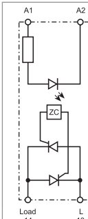
Schema semplificato
